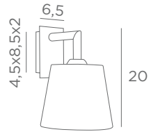
Lampshade EDFOU 1 o Ø 10-14-12 cm Lampshade code : 1125 + fabric code ↳ 16 cm
