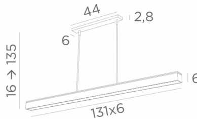
GALAND J tubes in geborsteld brons
