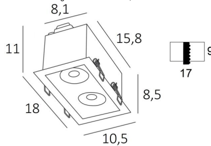
OURANOS 2 in gesatineerd chroom, zwart binnenkant
