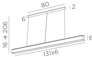
GALAND J # en laiton satiné. Finition du métal : code 25
