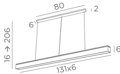
GALAND J # en laiton satiné. Finition du métal : code 25
