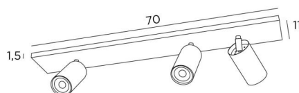
DEIMOS L2+1 en noir structuré et laiton satiné (code 45)
