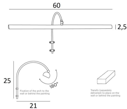
TRIANON 60 en nickel satiné. Finition du métal : code 33
