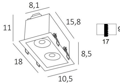
OURANOS 2 en laiton satiné. Finition du métal : code 25. Intérieur en noir structuré
