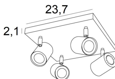
MAGELLAN SQUARE en bronze griffé. Finition du métal : code 29
