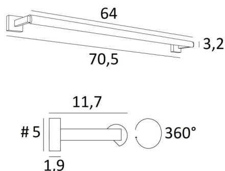
CREMONE 65 en bronze griffé. Finition du métal : code 29
