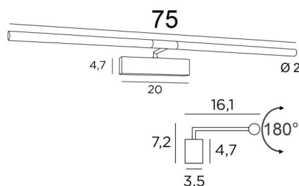
MEIDOUN 75 en nickel satiné. Finition du métal : code 33
